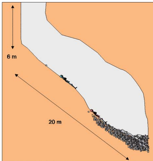
Fig. 2. Representación de la sima de Bedoña y localización de los restos. / Section and plan of Sima de Bedoña with the position of the remains.
