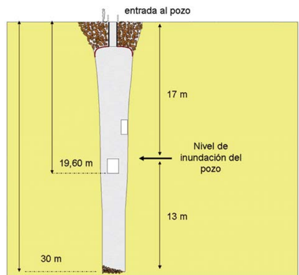
Fig. 12. Corte longitudinal del pozo El Salamanca Chico. / Section of El Salamanca Chico mine shaft.
